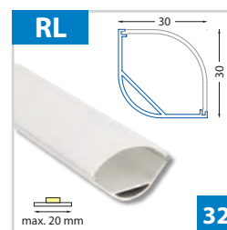
Rohový hliníkový profil 30x30 mm - pro pásy do šíře 20 mm
