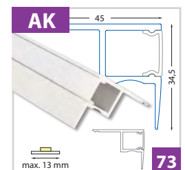
Podhledový hliníkový profil 45x35 mm - pro pásy do šíře 13 mm
