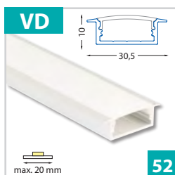
Vestavný hliníkový profil 31x10 mm - pro pásy do šíře 20 mm
