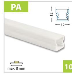
Přisazený PMMA profil 12x12 mm - pro pásy do šíře 8 mm
