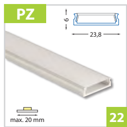
Přisazený hliníkový profil 24x6 mm - pro pásy do šíře 20 mm
