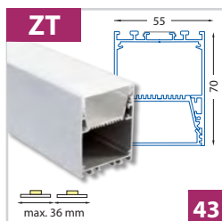
Závěsný hliníkový profil 55x70 mm - pro dva pásy do šíře 18 mm
