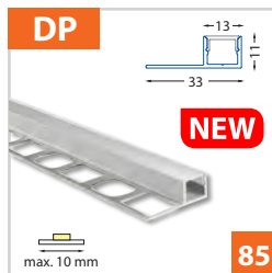
Obkladový hliníkový profil 33x11 mm - pro pásy do šíře 10 mm
