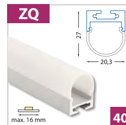
Závěsný hliníkový profil 20x27 mm - pro pásy do šíře 16 mm
