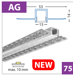
Vestavní hliníkový profil pro sádkarton 53x14 mm - pro pásy do šíře 10 mm
