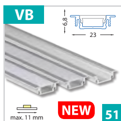
Vestavný hliníkový profil 23x7 mm - pro pásy do šíře 11 mm
