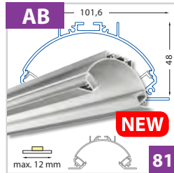
Podhledový hliníkový profil pro sádkarton 102x48 mm - pro pásy do šíře 12 mm
