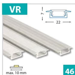
Vestavný hliníkový profil 22x7 mm - pro pásy do šíře 10 mm
