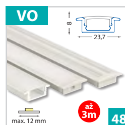
Vestavný hliníkový profil 24x8 mm - pro pásy do šíře 12 mm
