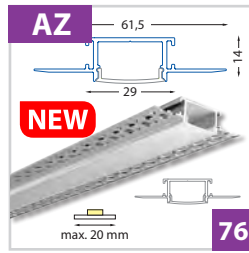
Vestavní hliníkový profil pro sádkarton 62x14 mm - pro pásy do šíře 20 mm
