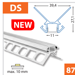
Obkladový hliníkový profil 39x27 mm - pro pásy do šíře 10 mm
