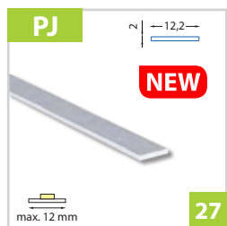
Přisazený hliníkový profil 12x2 mm - pro LED pásy do šíře 12 mm
