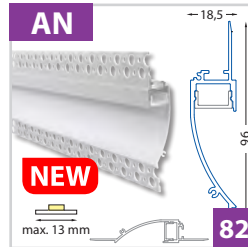
Vestavní hliníkový profil pro sádkarton 19x96 mm - pro pásy do šíře 13 mm
