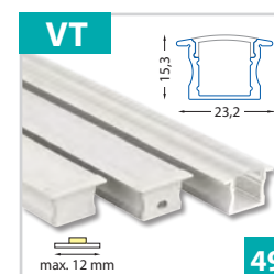
Vestavný hliníkový profil 23x15 mm - pro pásy do šíře 12 mm
