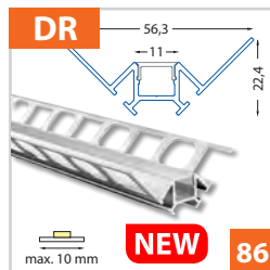
Obkladový hliníkový profil 56x22 mm - pro pásy do šíře 10 mm
