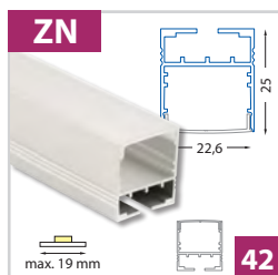
Závěsný hliníkový profil 23x25 mm - pro pásy do šíře 19 mm
