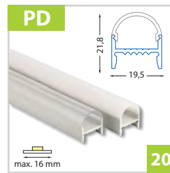
Přisazený hliníkový profil 20x22 mm - pro pásy do šíře 16 mm
