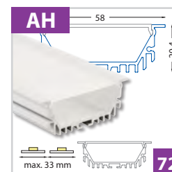
Vestavný hliníkový profil 58x20 mm - pro dva LED pásy do šíře 16 mm
