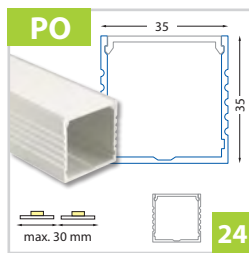
Přisazený hliníkový profil 35x35 mm - pro dva pásy do šíře 15 mm
