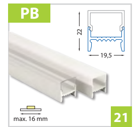
Přisazený hliníkový profil 20x22 mm - pro pásy do šíře 16 mm
