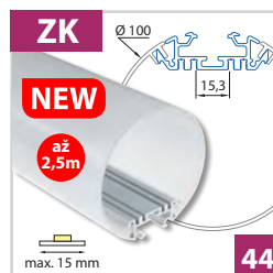
Závěsný hliníkový profil Ø 100 mm - pro pásy do šíře 15 mm
