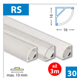
Rohový hliníkový profil 16x16 mm - pro pásy do šíře 10 mm
