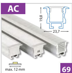
Vestavný hliníkový profil 24x20 mm - pro pásy do šíře 12 mm
