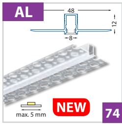
Vestavní hliníkový profil pro sádkarton 48x12 mm - pro pásy do šíře 5 mm
