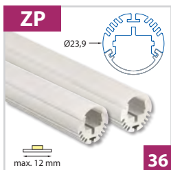
Závěsný kruhový hliníkový profil Ø 24 mm - pro pásy do šíře 12 mm
