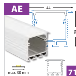
Vestavný hliníkový profil 44x35 mm - pro pásy do šíře 30 mm
