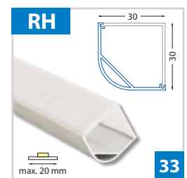
Rohový hliníkový profil 30x30 mm - pro pásy do šíře 20 mm
