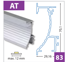
Vestavní hliníkový profil pro sádkarton 29x70 mm - pro pásy do šíře 12 mm
