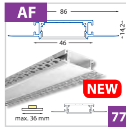
Vestavní hliníkový profil pro sádkarton 88x19 mm - pro pásy do šíře 36 mm
