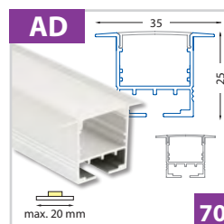
Vestavný hliníkový profil 35x25 mm - pro pásy do šíře 20 mm
