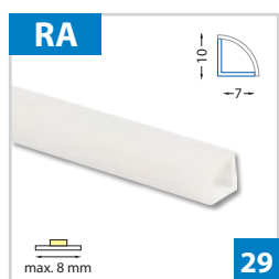
Rohový PMMA profil 7x10 mm - pro pásy do šíře 8 mm
