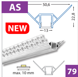
Rohový hliníkový profil pro sádkarton 51x23 mm - pro pásy do šíře 10 mm
