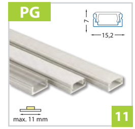
Přisazený hliníkový profil 15x7 mm - pro pásy do šíře 11 mm
