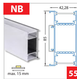
Nástěnný hliníkový profil 42x85 mm - pro pásy do šíře 15 mm
