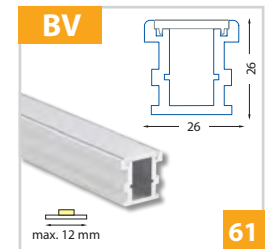
Nášlapný hliníkový profil 26x26 mm - pro pásy do šíře 12 mm
