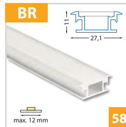
Nášlapný hliníkový profil 27x11 mm - pro pásy do šíře 12 mm
