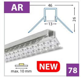
Rohový hliníkový profil pro sádkarton 46x26 mm - pro pásy do šíře 10 mm
