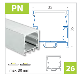
Přisazený hliníkový profil 35x35 mm - pro dva pásy do šíře 12 mm
