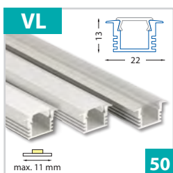
Vestavný hliníkový profil 22x13 mm - pro pásy do šíře 11 mm
