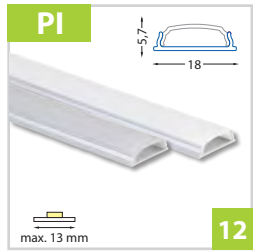
Přisazený hliníkový profil 18x6 mm, ohebný - pro pásy do šíře 13 mm
